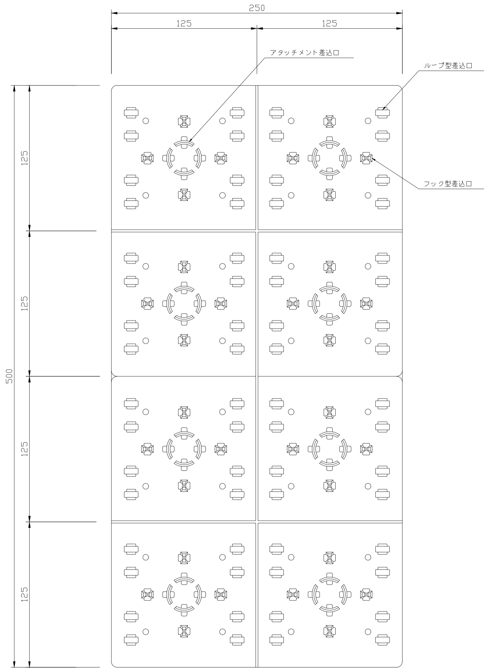
デコプラ基盤平面図
