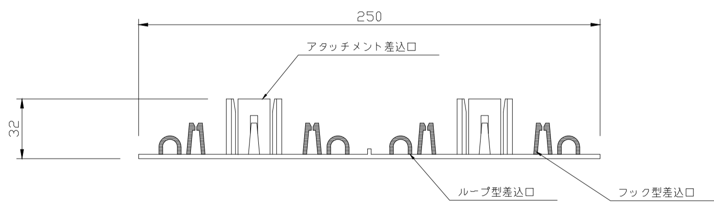
デコプラ基盤側面図
