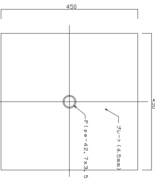
組立詳細図 1/8
