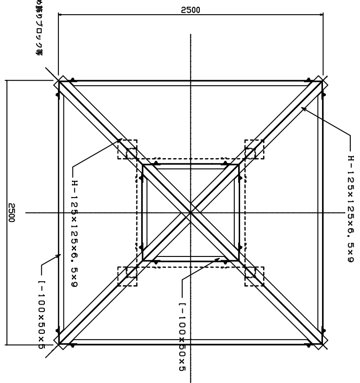
基礎図 1/25
